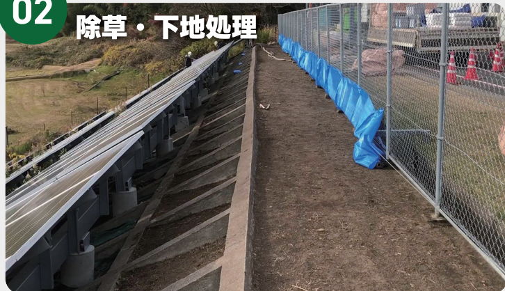
除草後に地盤や法面の下処理を行う。
