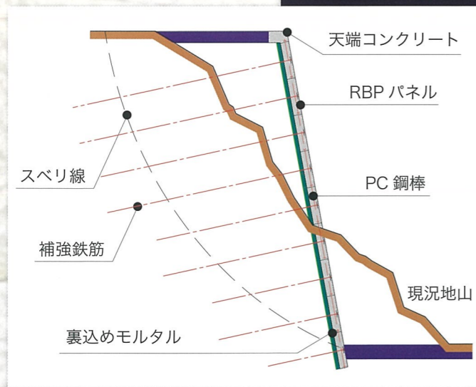
■参考断面図
